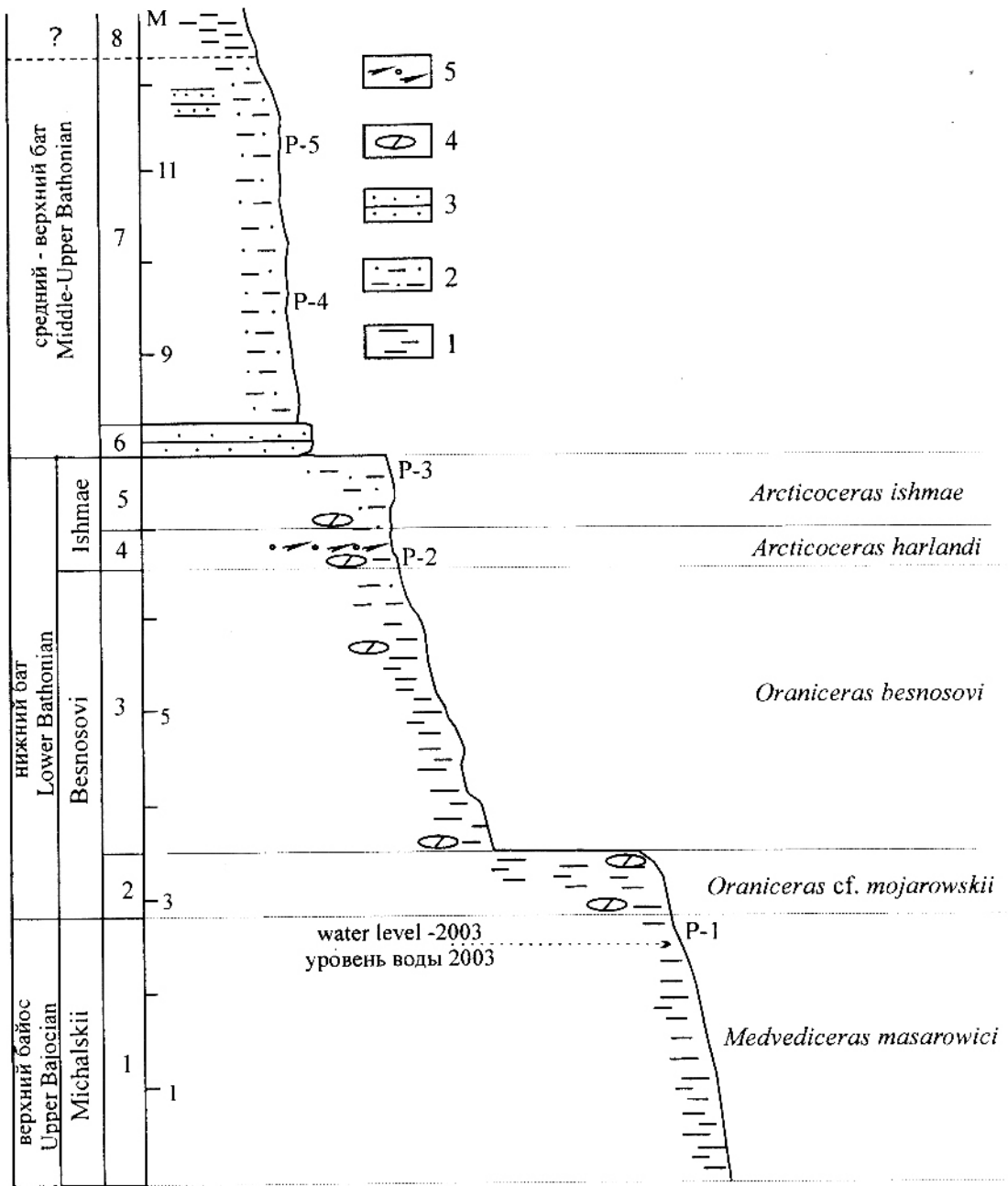
Рис. 2. Разрез в карьере "Сокурский". Условные обозначения: 1- глина; 2- алеврит; 3- алевролит; 4- сидеритизированные стяжения, 5- "белемнитовый уровень", P-1-5- уровни отбора палинологических образцов. Шкала линейки 1 м.
