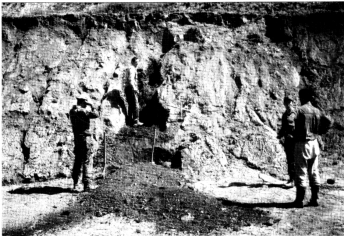
Рис. 1. Средний уступ карьера "Сокурский" в окрестностях г. Саратов. Фото Й. Грюнделя, 2003 г.
